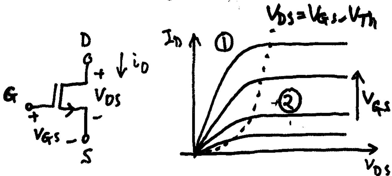
n-channel enhancement-mode MOSFET
